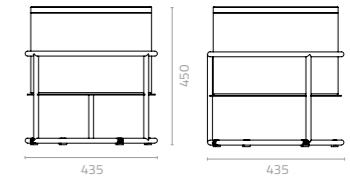
Ollo stool W435x D435 x H450mm Packing: 0.104m 3 , 1pc/ctn
